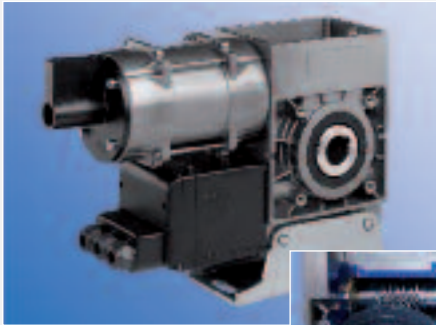
Aufsteckantrieb TAR mit integrierter Fangvorrichtung.
